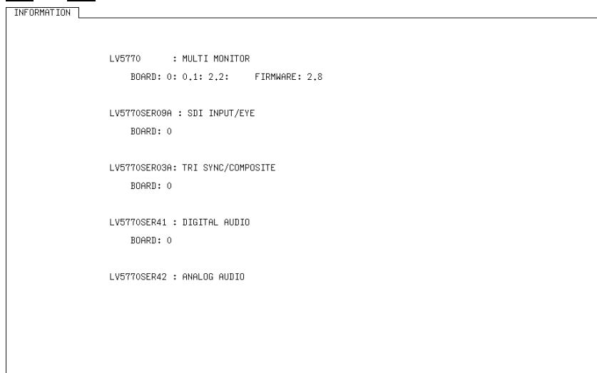
図 7-8 INFORMATION 画面
